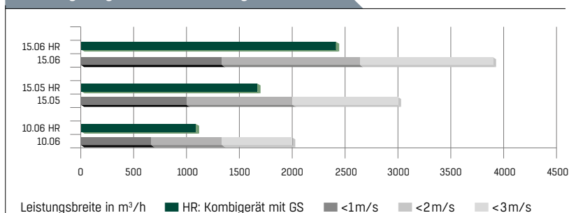
Leistungsdiagramm der drei Baugrößen
